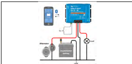
Figure 1 : Branchement typique en tant que convertisseur CC-CC
