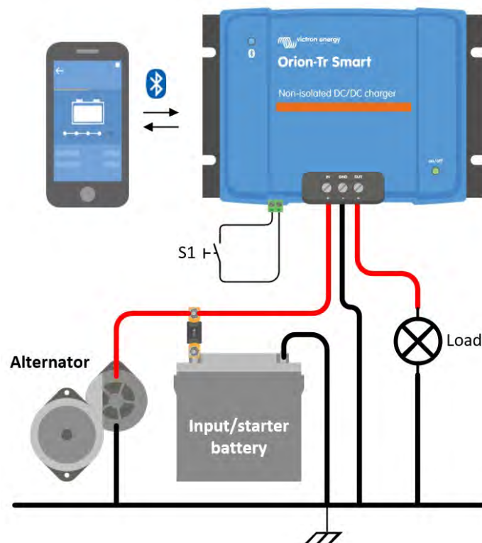
Abbildung 1: Typischer Verbindungsaufbau als DC-DC-Wandler
