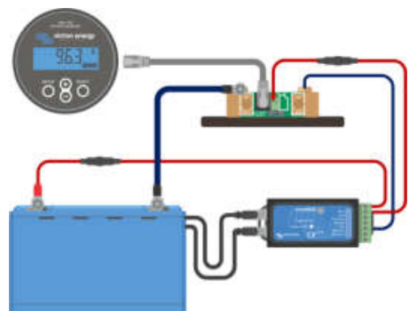
Das Stromkabel des Batteriemonitors ist mit dem BMS verbunden
