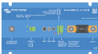
Das Smart BMS CL 12/100
