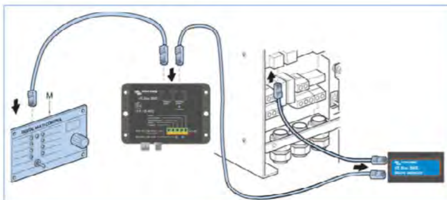
Bild 4: VE.Bus-anslutningar
