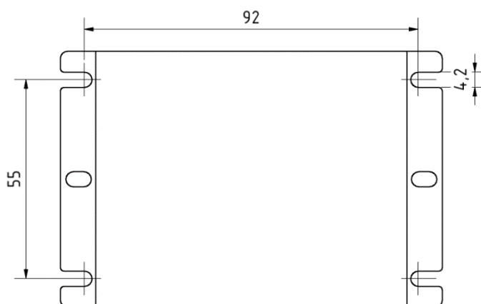
Abbildung 2: Abmessungen der Anschraubpunkte des Gehäuses
