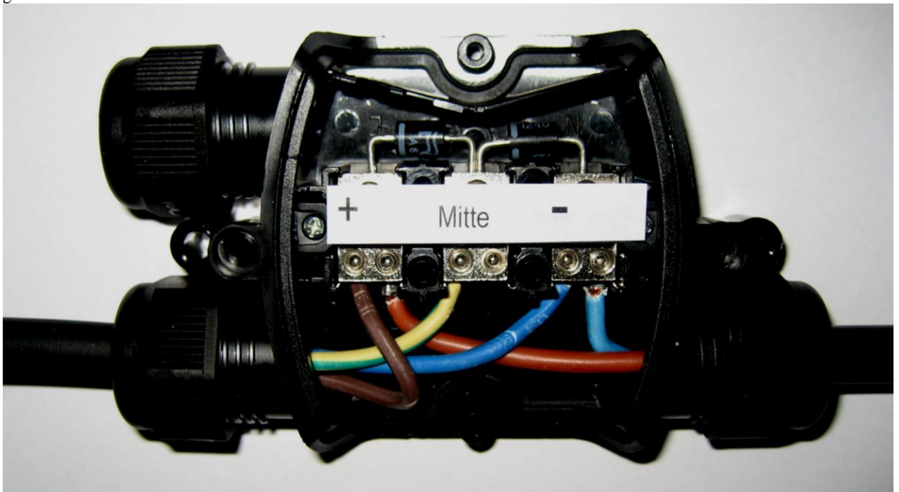
Abbildung : Links wird das dreidrigige Solarkabel des Solarmoduls in die Diodenbox eingeführt (Farbe: Braun, Gelb, Blau); Rechts wird das Kabel zum Laderegler aus der Diodenbox herausgeführt
